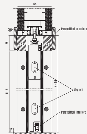
Sezione verticale
