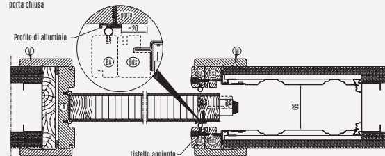
Sezione orizzontale porta chiusa
