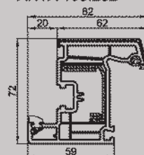
ANTA 103.232
