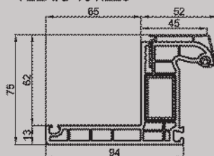
TELAIO 101.229
