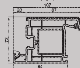
ANTA MAGGIORATA 103.241
