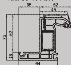
TELAIO 101.219
