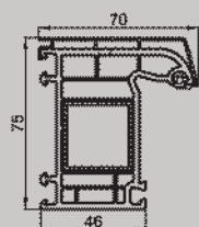
TELAIO 101.233
