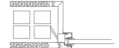
APPLICAZIONE PER MURATURA APPLICATION ON BRICKWORK
