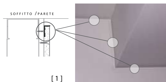
Bf per realizzare fughe parete | soffitto Bf to make wall - ceiling channel
