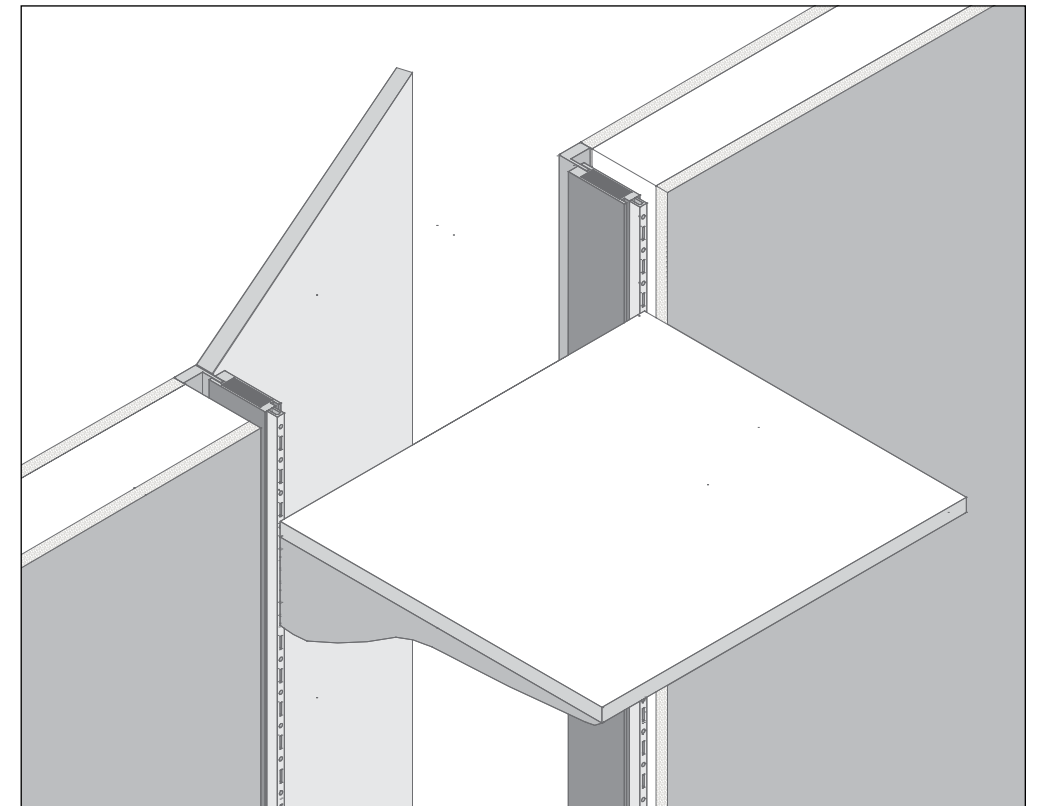
Dettaglio dell'aggancio della cremagliera sul profilo Fil Zero Detail of hooking up the rack to the Fil Zero Profile
