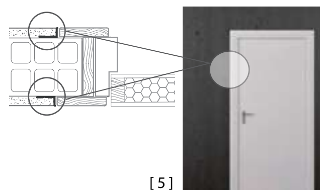
Bf per incassare a filo le cornici delle porte Bf to recess the trim flush wall
