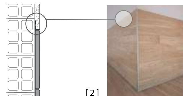
Bf per inserimento rivestimenti a parete (es. piastrelle, doghe, etc.) Bf for inserting wall claddings (tiles, planks etc)
