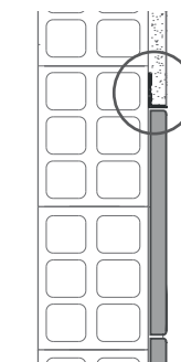
Bf per fare il filo tra il rivestimento delle piastrelle, doghe o altro rivestimento di spessore e la parete ed evitare cornici e listelli di finitura. Bf for filling the grouting between the coating, tiles, slats or other veneer thicknesses and the wall, thus avoiding any finishing frames or strips.
