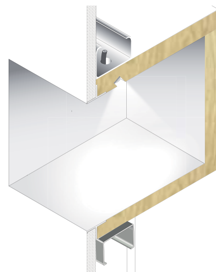
Ob light inserito nella struttura OPEN BOX INSERTED IN THE STRUCTURE
