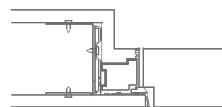
APPLICAZIONE PER CARTONGESSO APPLICATION ON PLASTERBOARD
