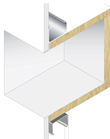
Open Box inserito nella struttura OPEN BOX INSERTED IN THE STRUCTURE
