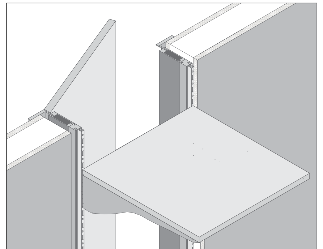
Dettaglio dell'aggancio della cremagliera sul profilo Fill Out Detail of hooking up the rack to the Fill Out Profile
