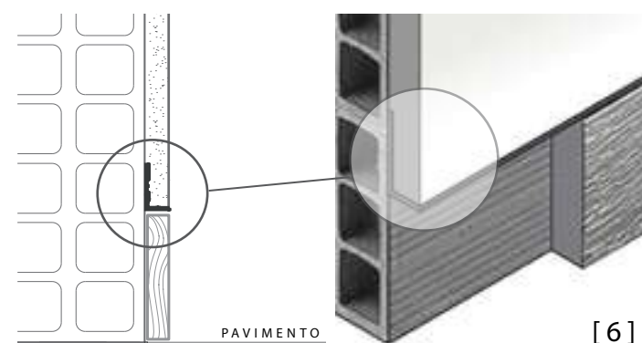
Bf per incassare il battiscopa Bf to recess the skirting board
