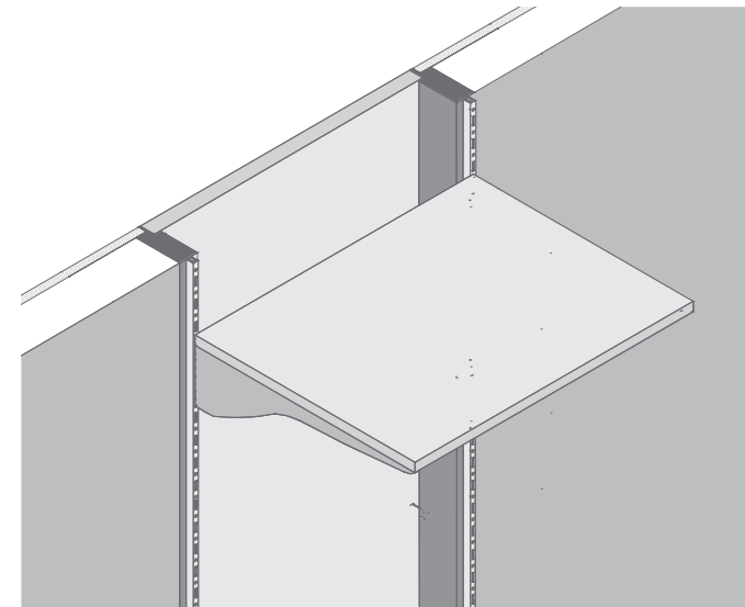
Dettaglio dell'aggancio della cremagliera sul profilo fantasmينو.
