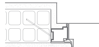
APPLICAZIONE PER MURATURA APPLICATION ON BRICKWORK
