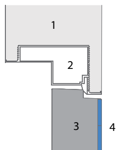
PORTE A SPINGERE | PUSH DOOR
