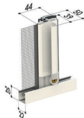
Barra maniglia doppia
