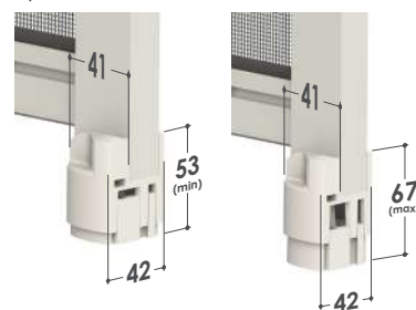
Piedini ad espansione di serie, apertura massima
