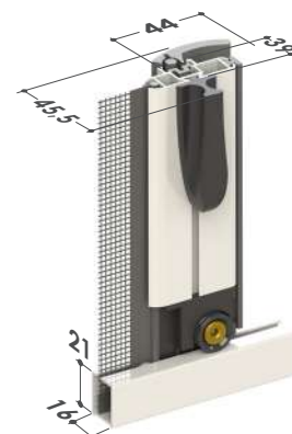
Cassonetto da 50 Testate inferiori
