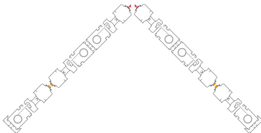
ANTA DOPPIA CON APERTURA BILATERALE ANGOLARE
