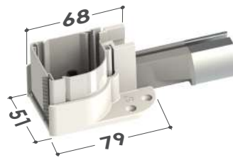
Cassonetto da 45 Testate inferiori
