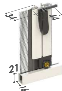
Cassonetto da 50 Testate inferiori
